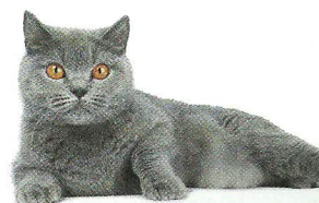
8 chat/panthère/sauvage
