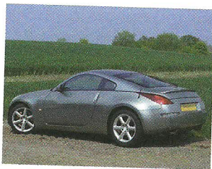
2 voiture/scooter/cher
